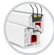
T-Energy 6 camere profondità del telaio 88 mm
